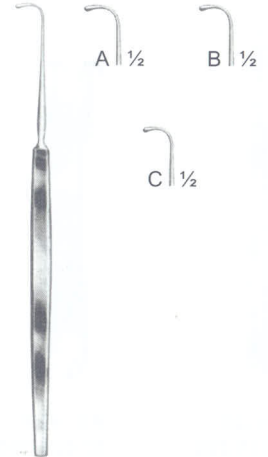
GRAEFE 07-044-130 13.0 cm - A 07-045-140 14.0 cm - B 07-046-150 15.0 cm - C
