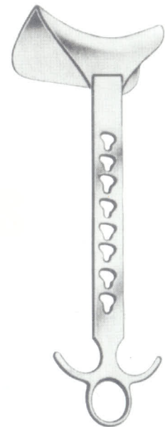
ROCHARD 07-530-310 31 cm 48 mm x 90 mm 07-531-310 31 cm 48 mm x 105 mm 07-532-310 31 cm 48 mm x 120 mm 07-533-310 31 cm 48 mm x 135 mm 07-534-310 31 cm 48 mm x 155 mm
